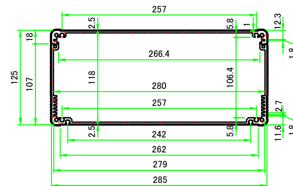
A-A (1:5)
